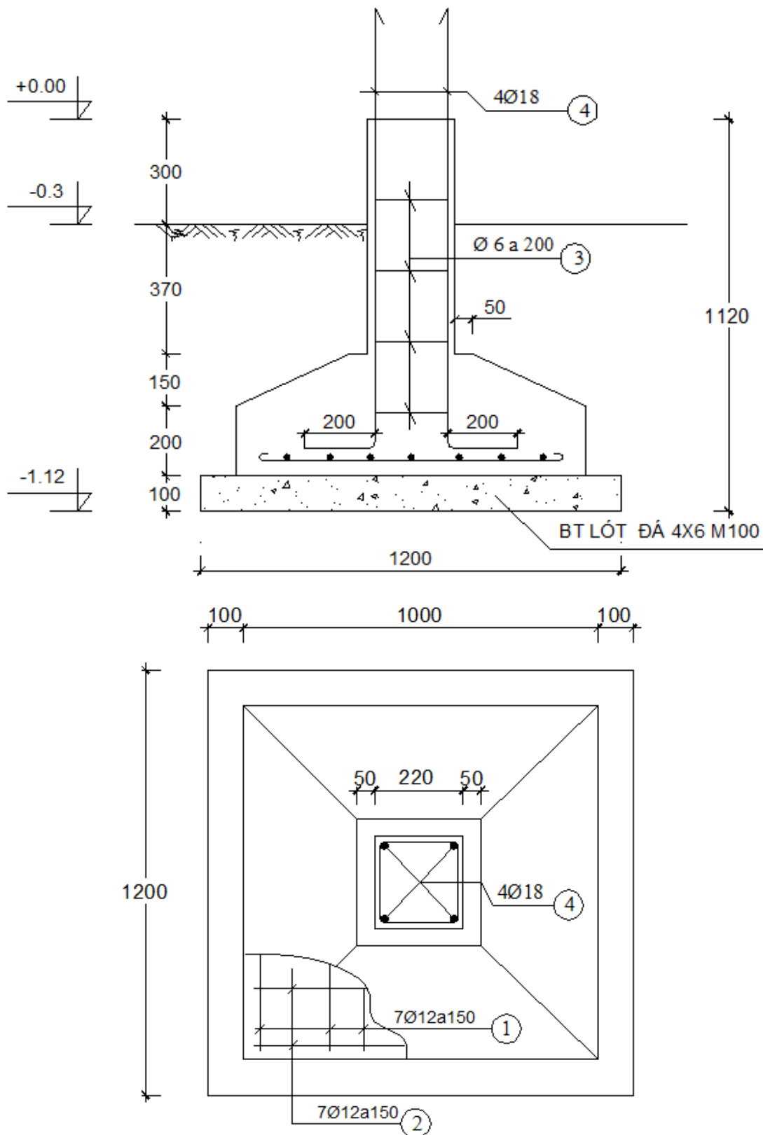
Móng M1
