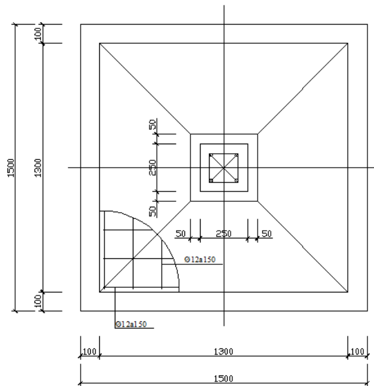
MÓNG M1
