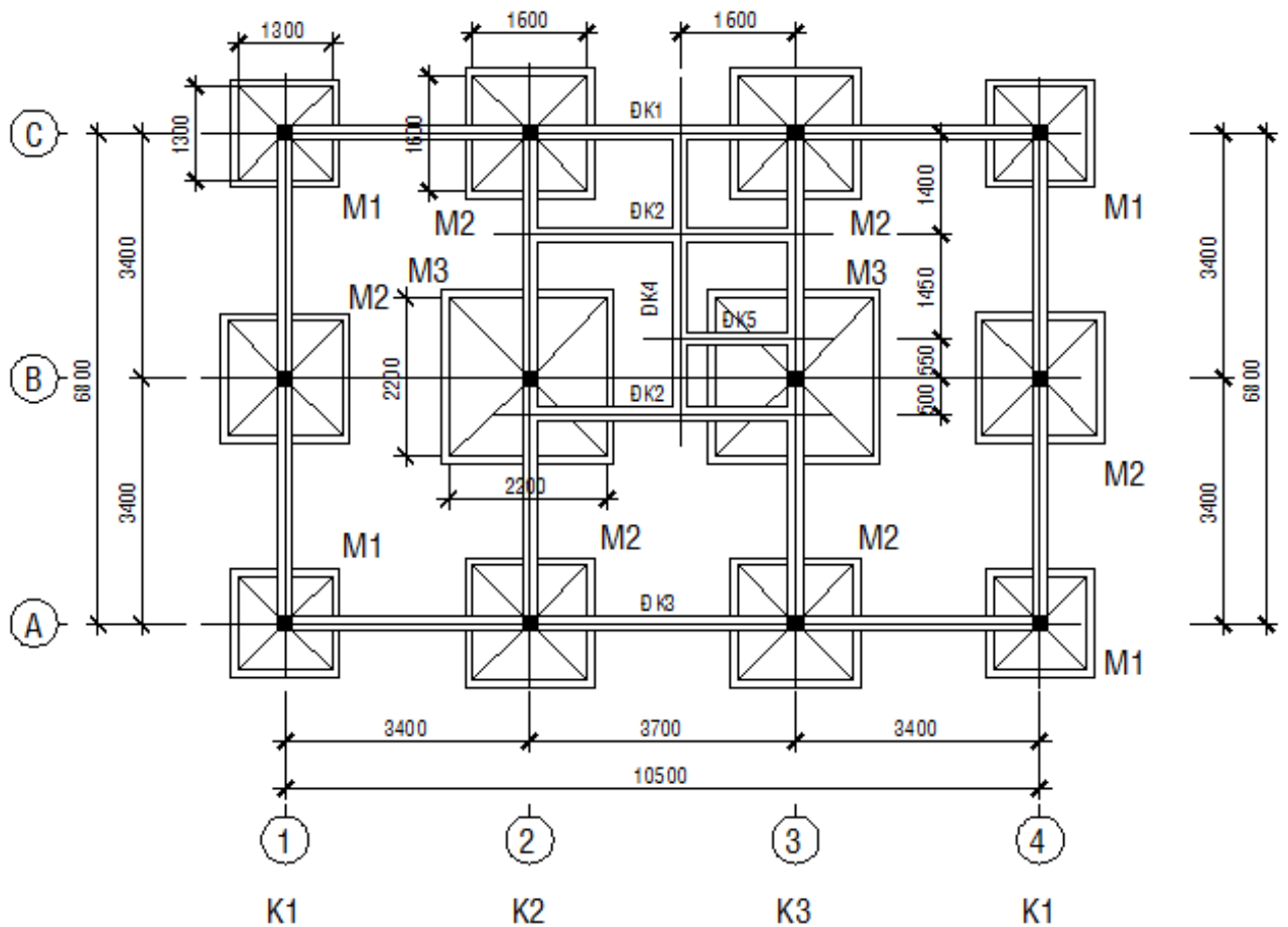
MẶT BẰNG MÓNG TL : 1/100
